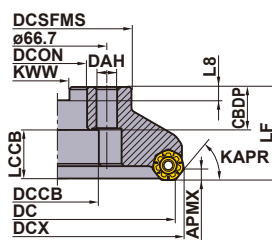
Şek. 3 ø160
