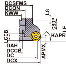
Şek.1 ø80
