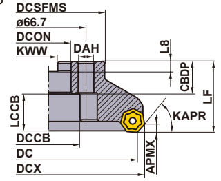
Şek.3 ø160
