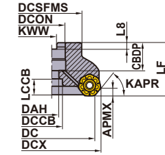
Şek. 1 ø63 ø80
